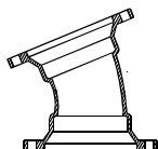
BENDS : MJ X MJ 22½° (1/16)
