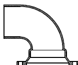
BENDS : MJ X PE 90° (1/4)
