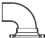
BENDS : MJ X PE 90° (1/4)
