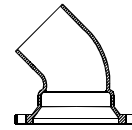
BENDS : MJ X PE 45° (1/8)
