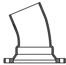
BENDS : MJ X PE 22½° (1/16)
