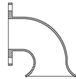
90° FLANGE X FLARE BENDS
