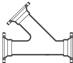
MJ 45° LATERAL (WYES)
