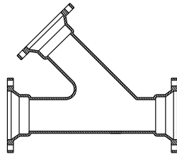
MJ 45° LATERAL (WYES)
