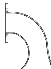
LONG RADIUS 90° FLANGE X FLARE BENDS
